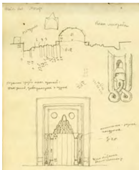
Рис. 6. План, фасад и вид фрагмента михраба. Кроки, 1928 г. Автор не установлен, предположительно – Б. Н. Засыпкин [по: 10, с. 380, рис. 7]
