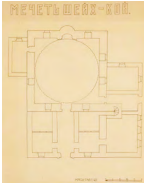
Рис. 7. План мечети в селении Шейх-Кой. Автор – предположительно Б. Н. Засыпкин. 20-е гг. XX в. (ЦГАЛИ. Ф. Р-598. Оп. 1. Д. 493. Л. 14)
